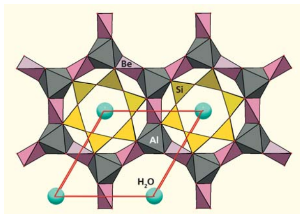
Рис.2. Структура берилла.
