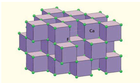
Рис. 11. Структура флюорита.
