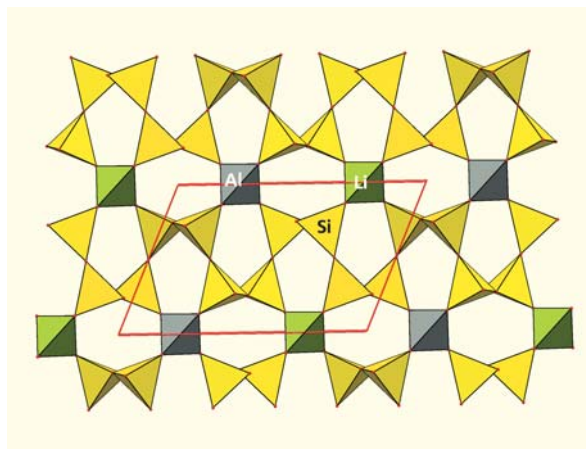
Рис.6. Структура петалита.
