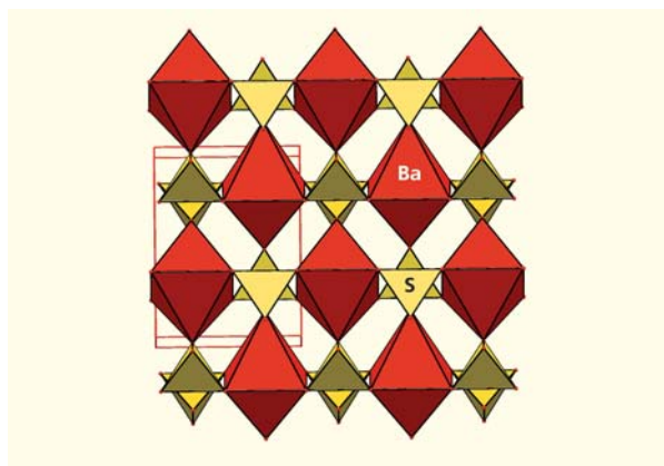
Рис.1. Структура барита.
