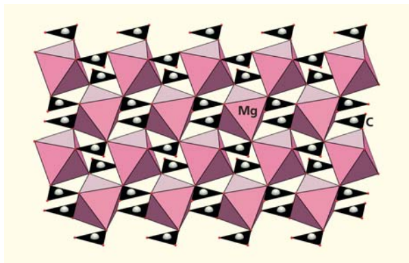
Рис.7. Структура магнезита.
