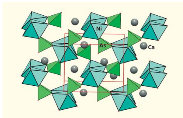
Рис.8. Структура никельаустинита.
