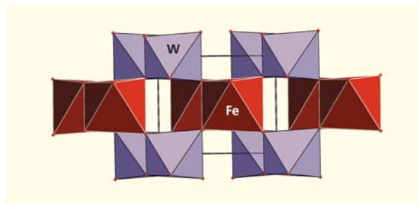
Рис.4. Структура ферберита.
