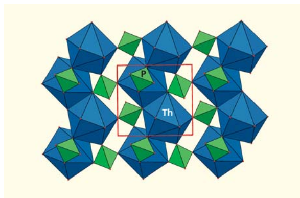
Рис.10. Структура монацита.
