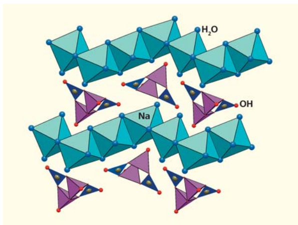
Рис.3. Структура буры.
