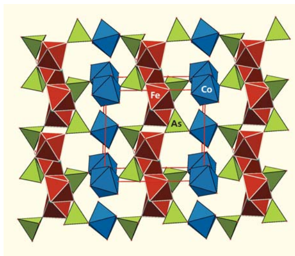
Рис.5. Структура кобальтартурита.
