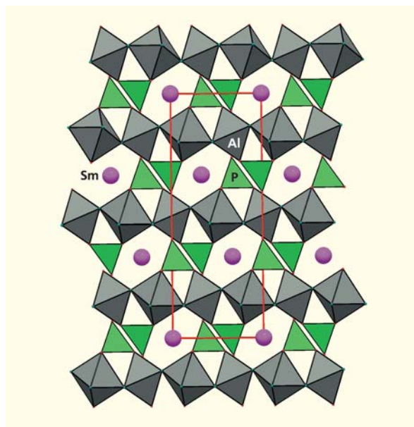
Рис.9. Структура флоренсита-(Sm).
